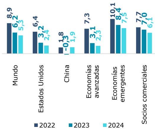
Gráfico 1.2. Inflación y crecimiento del PIB global (%)
